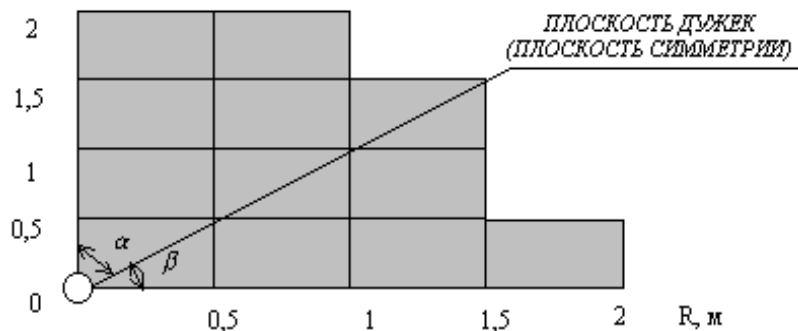
Рис. 9. Схема расположения мерных банок при испытании пенных оросителей:
