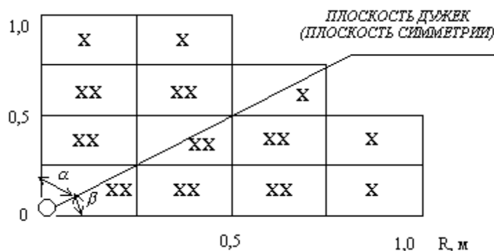
Рис. 4. Схема расположения мерных банок при испытании оросителей для стеллажных складов с d_y=10 и 12 мм:
